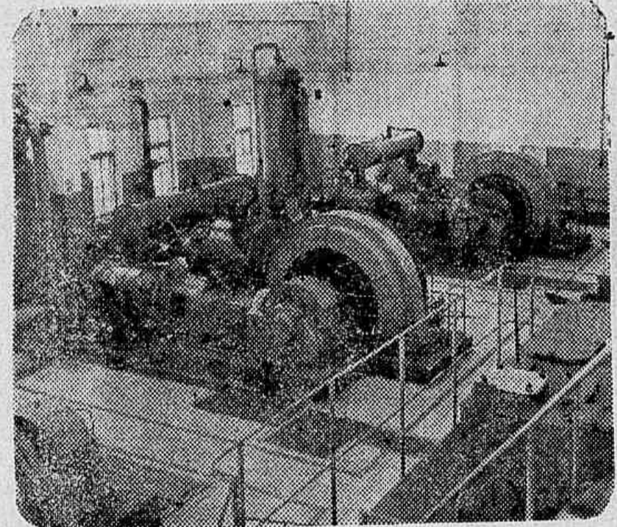
A estação elétrica de Shatsk é movida a turbina de gás. O seu combustível procede da gasificação subterrânea do carvão. A foto mostra três poderosas máquinas que suprem de ar os geradores subterrâneos de gás (Foto TASS)
