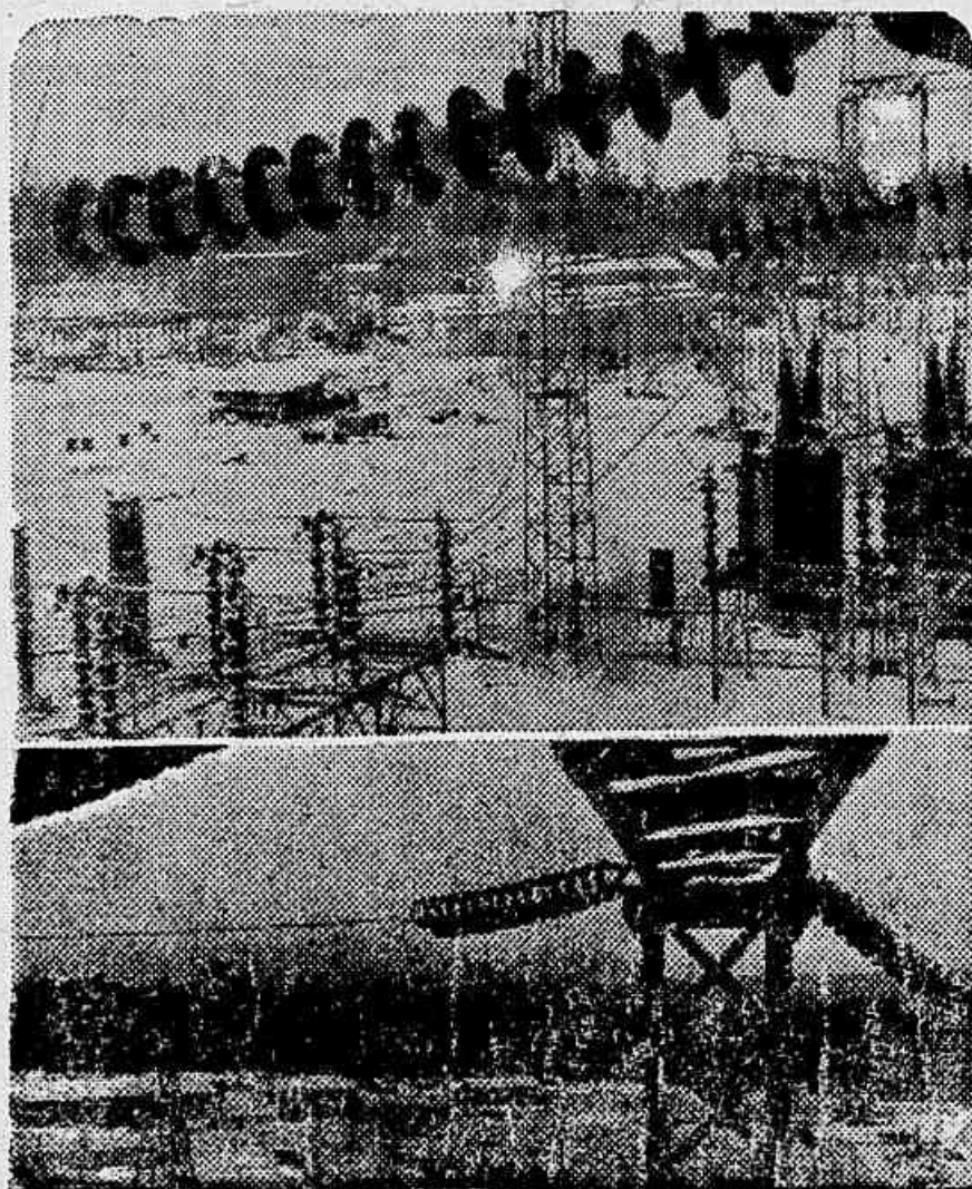
Prosegue a construção da hidrelétrica, de Bratsk, na Sibéria, que deverá ter 3.200.000 de Kws de potência, virão a ser, assim, a maior hidrelétrica do mundo. Vemos, no clichê, dois aspectos da sub-estação de abaixamento, construída num setor da linha Irkutsk-Bratsk. Todo um sistema de sub-estações servirá à indústria daquela região. (Foto TASS)
