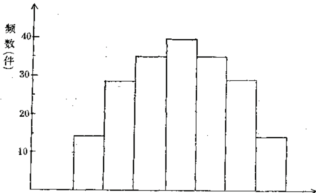
直 方 图
