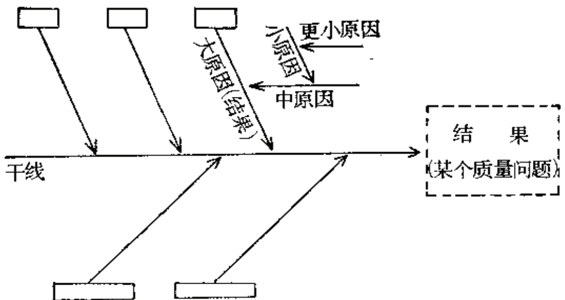
因果图
